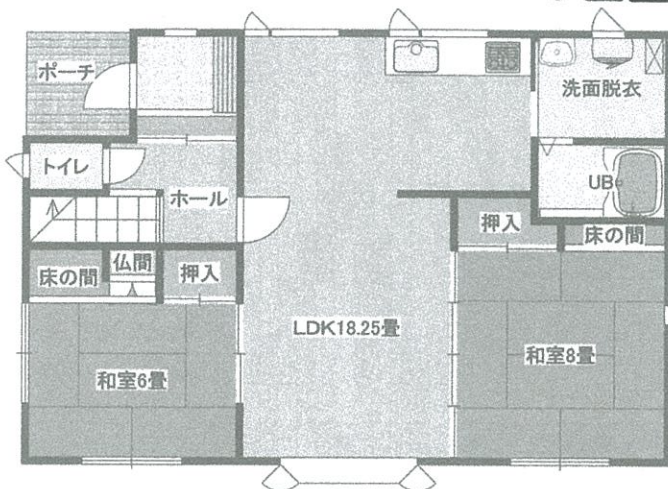
1階 平面図
