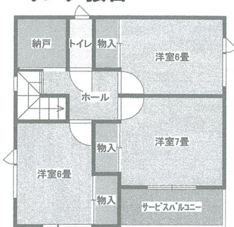
2階 平面図
