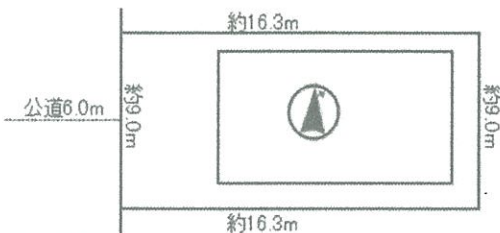
敷地配置図
