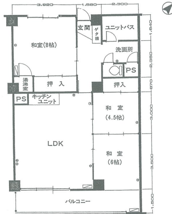
■ 間取図 ■
